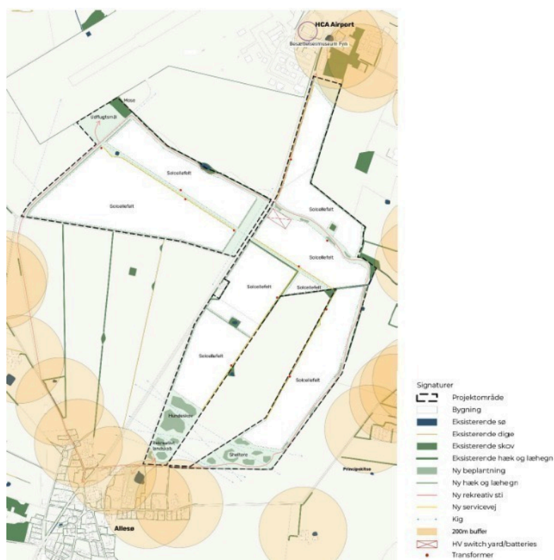
Figur 2: Principskitse for solenergianlægget.
